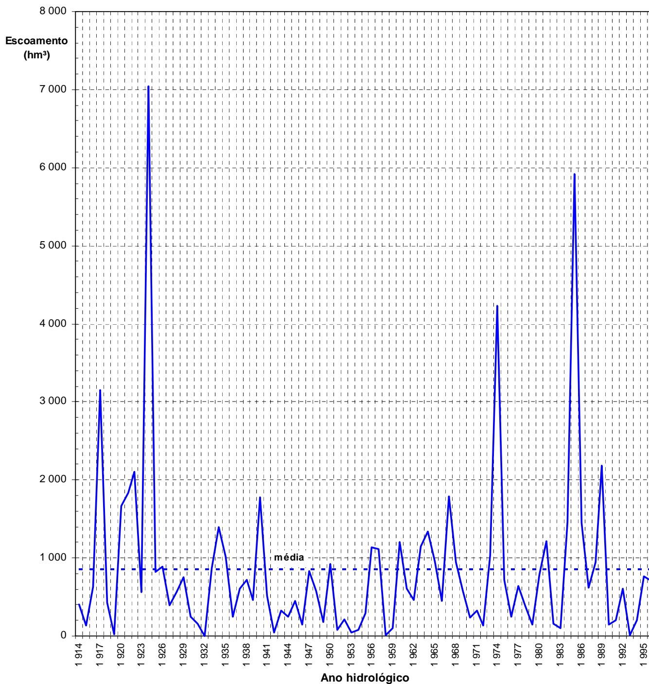
Figura 3.1 Açude Orós - Série de escoamentos anuais
